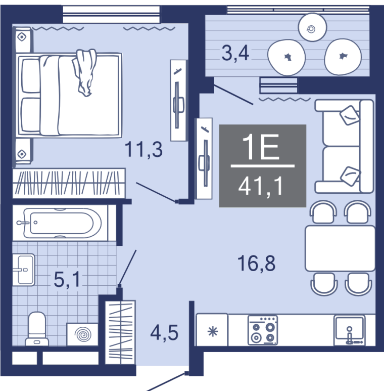
План этажа
