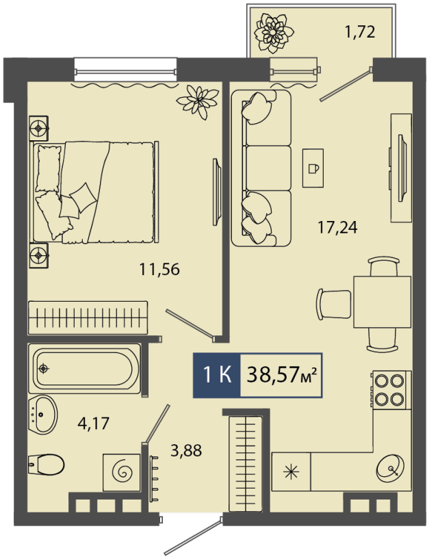
План этажа
